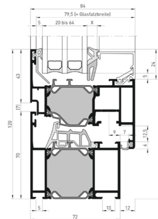
Schnittdarstellung BLECHER Alu W 72
